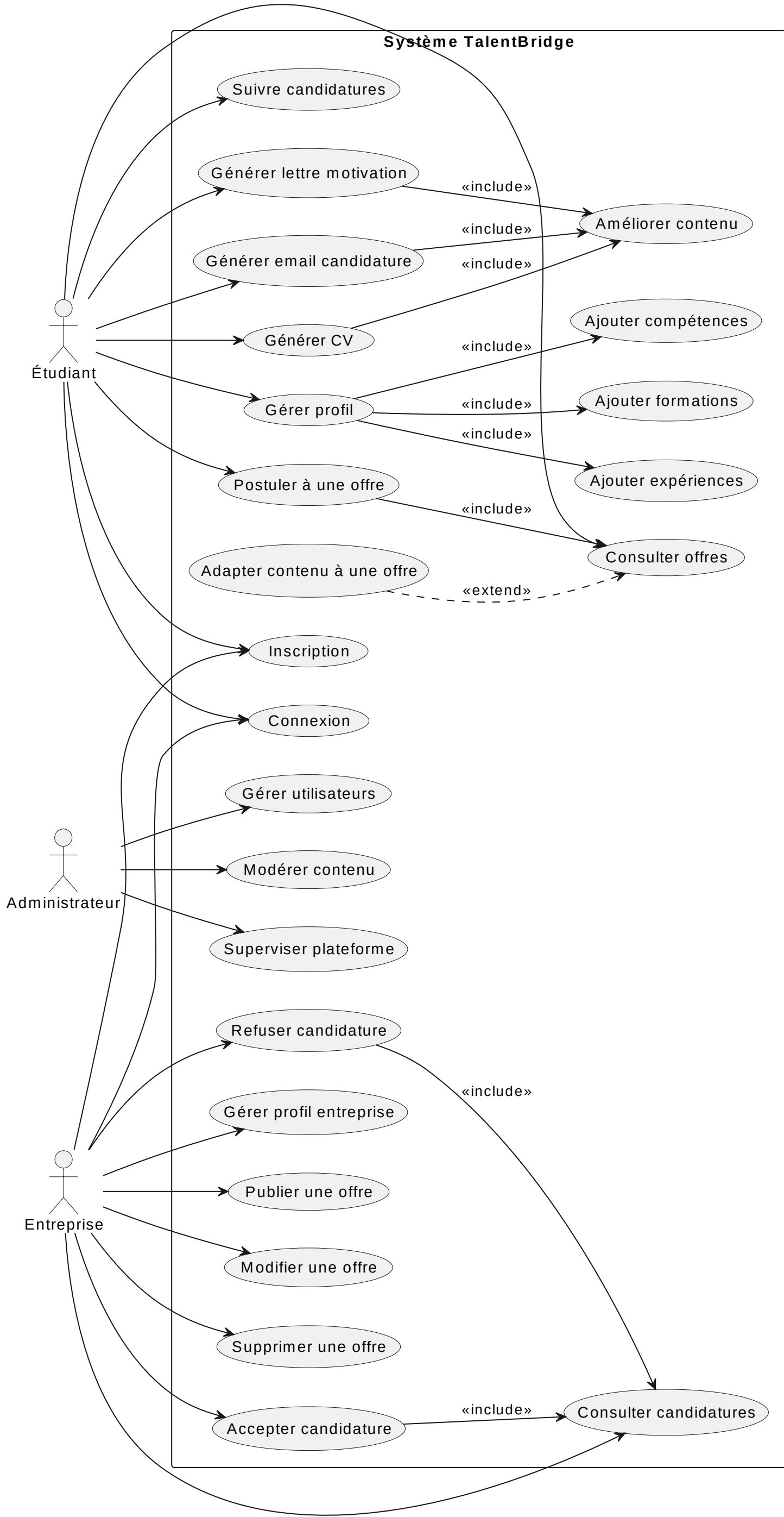
Diagramme de Cas d'Utilisation - TalentBridge + IA (Version Avancée)
